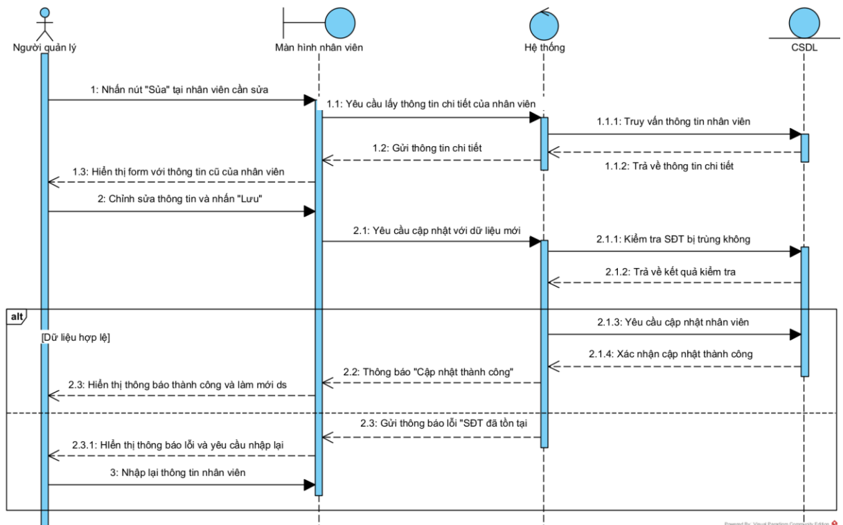
Hình 3.52. Biểu đồ tuần tự chức năng Sửa thông tin nhân viên
