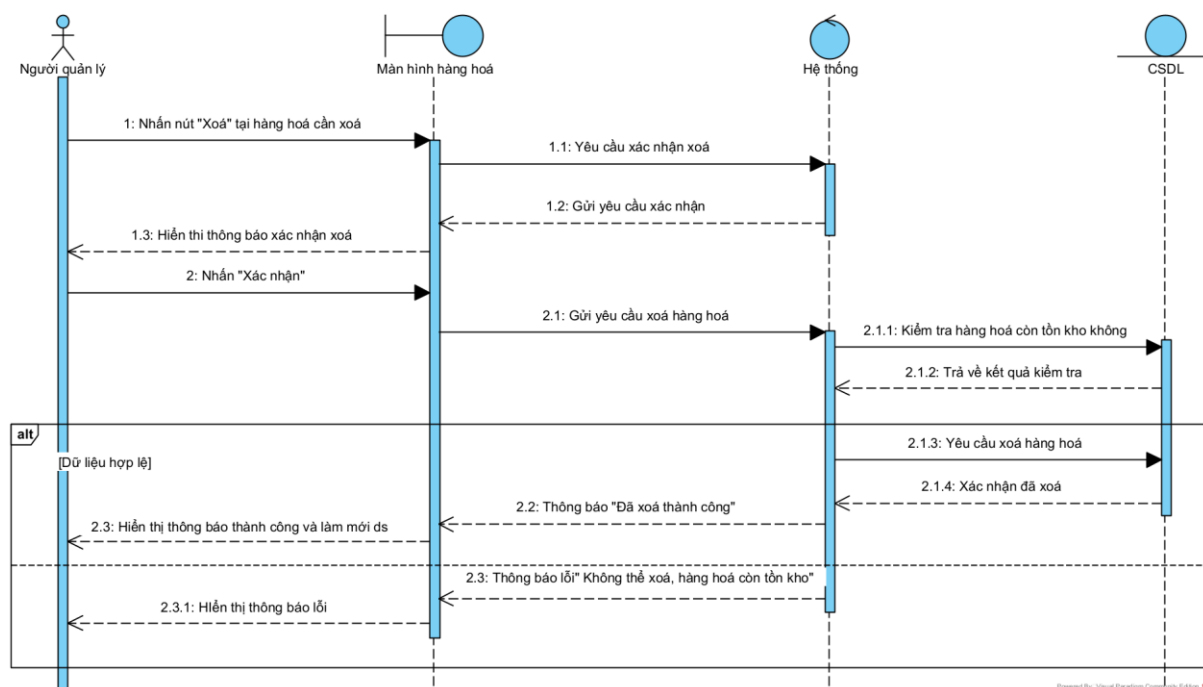
Hình 3.50. Biểu đồ tuần tự chức năng Xóa hàng hóa
