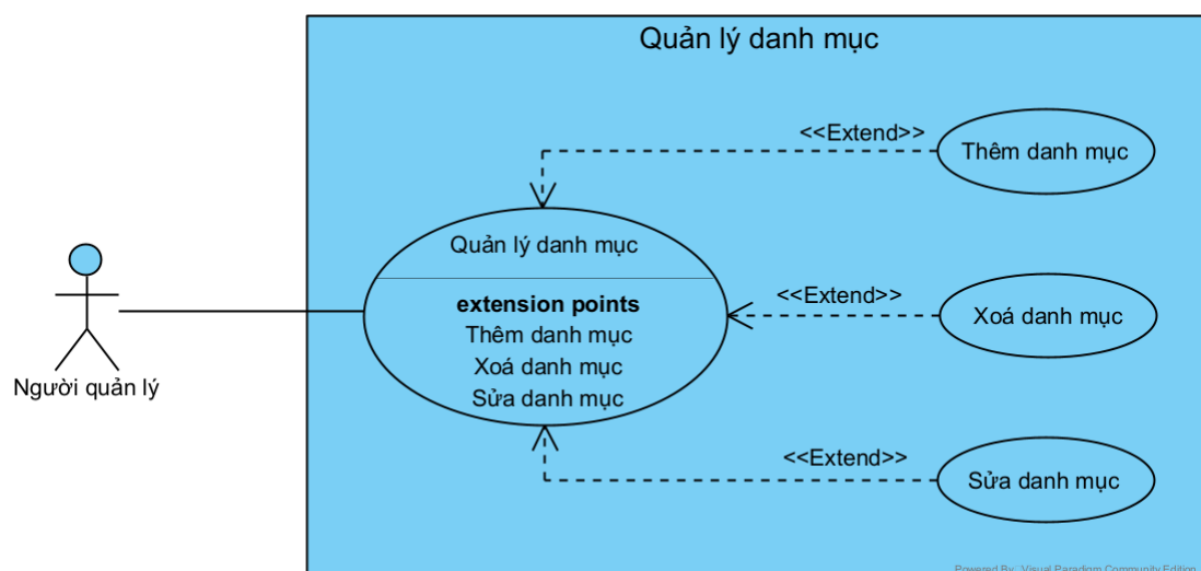
Hình 3.12. Biểu đồ UC mức 3 Quản lý danh mục
