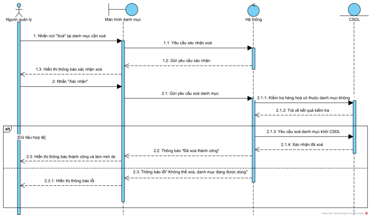
Hình 3.47. Biểu đồ tuần tự chức năng Xóa danh mục ngành hàng
