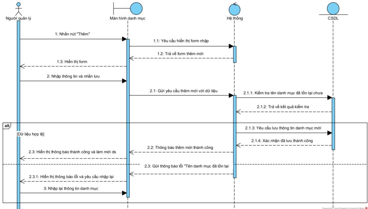
Hình 3.45. Biểu đồ tuần tự chức năng Thêm danh mục Ngành hàng
