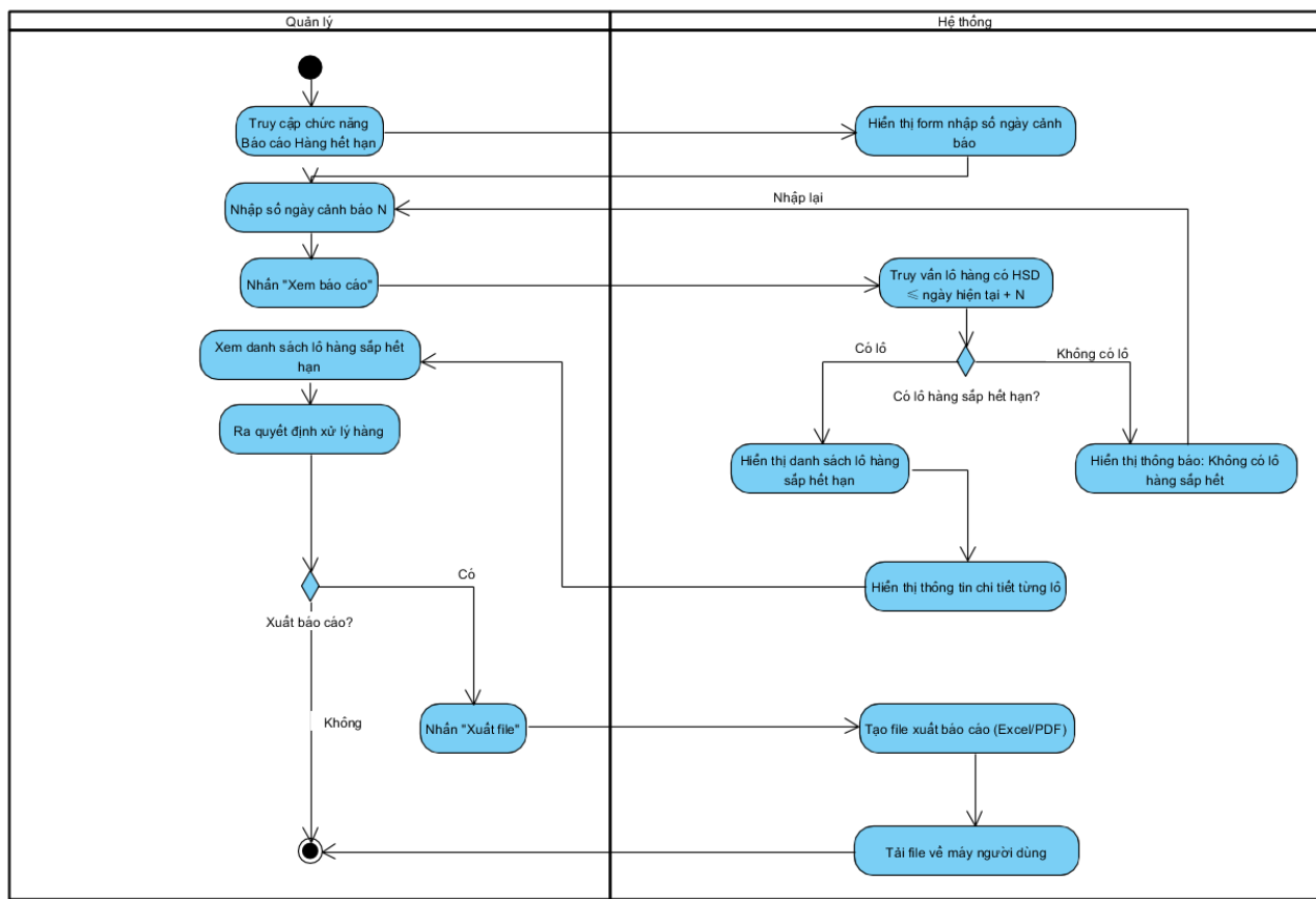
Hình 3.23. Biểu đồ Activity Báo cáo hàng hết hạn
