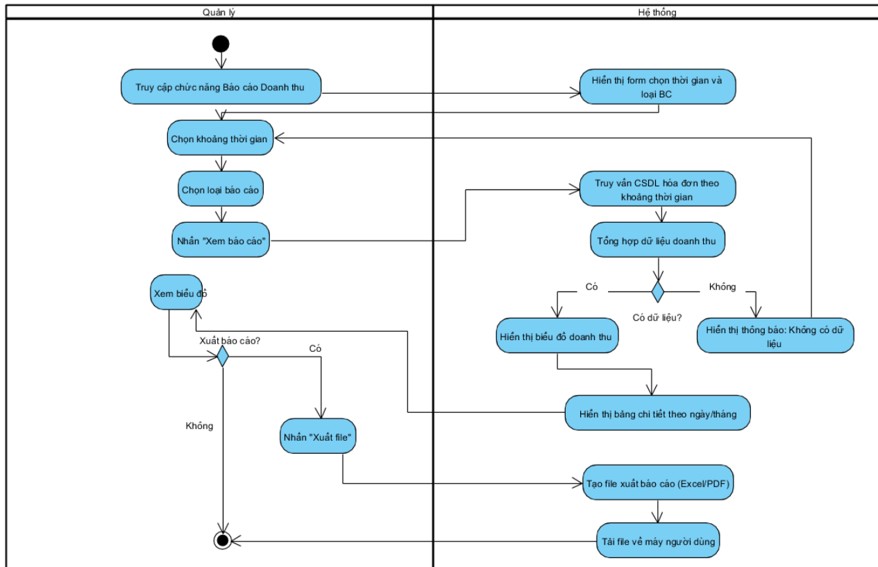
Hình 3.22. Biểu đồ Activity Báo cáo doanh thu
