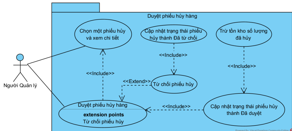
Hình 3.10. Biểu đồ UC mức 3 Duyệt phiếu hủy hàng
