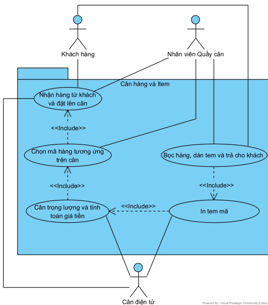
Hình 3.4. Biểu đồ UC mức 3 Cân hàng và In tem
