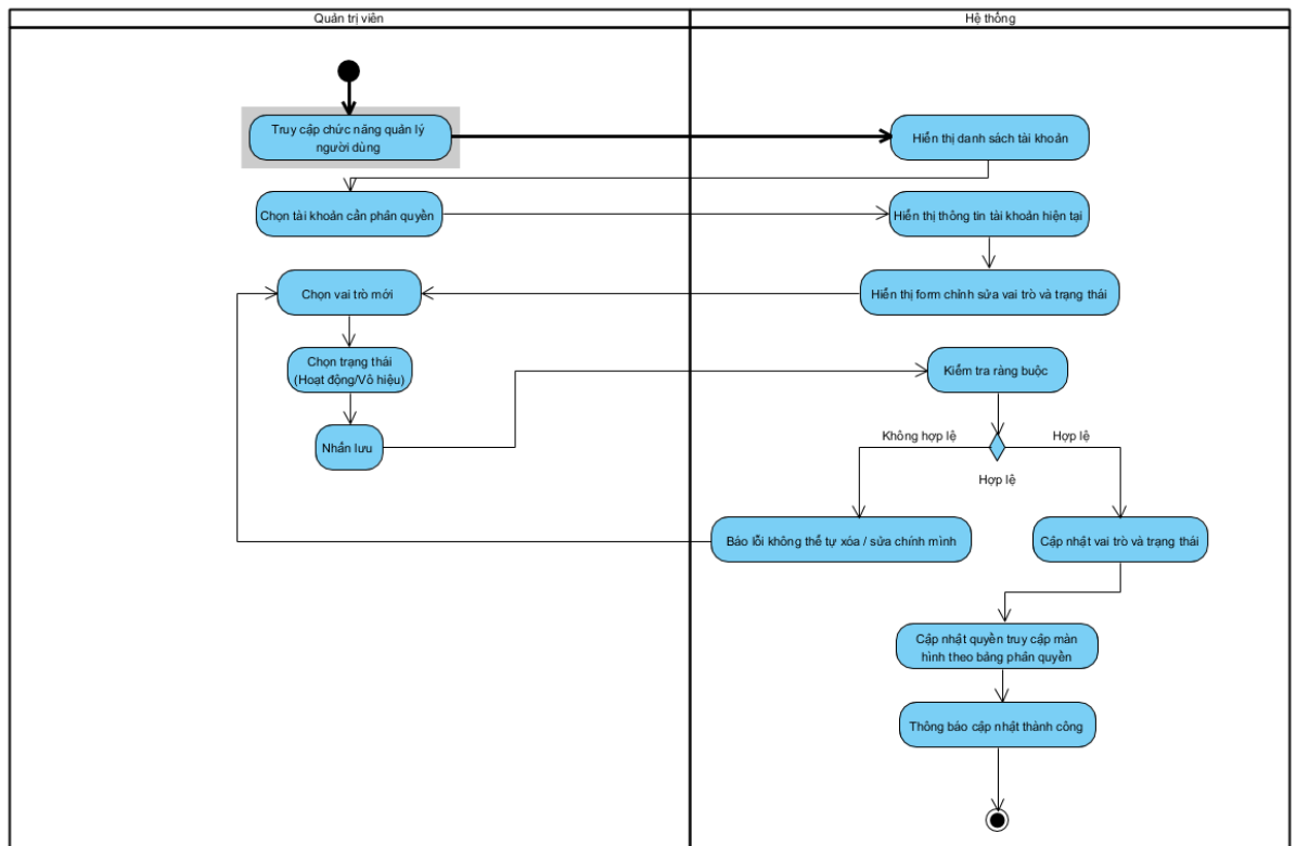
Hình 3.19. Biểu đồ Activity Phân quyền
