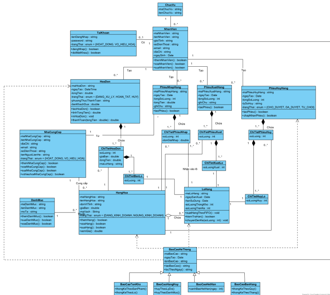
Hình 3.34. Biểu đồ Class
