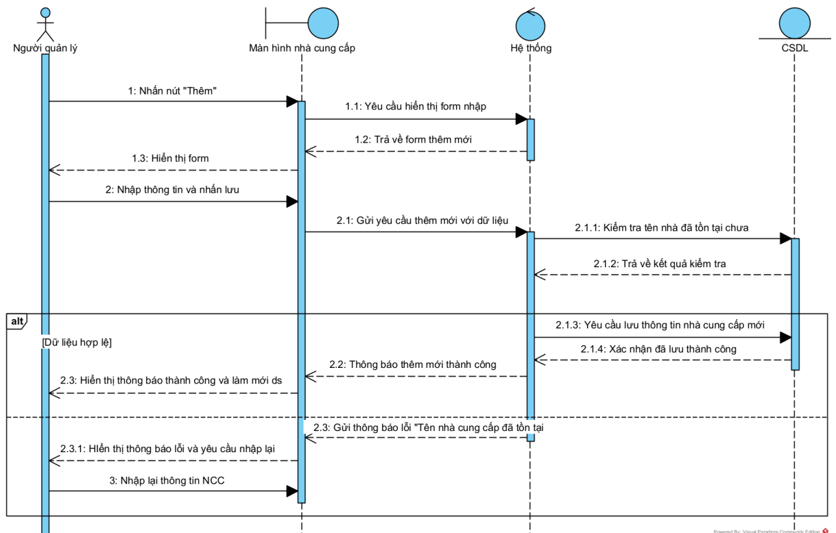
Hình 3.54. Biểu đồ tuần tự chức năng Thêm mới nhà cung cấp
