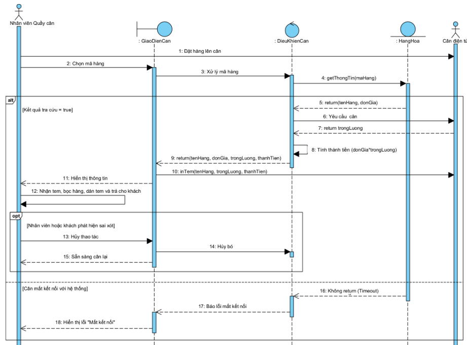
Hình 3.39. Biểu đồ tuần tự chức năng Cân hàng và In tem
