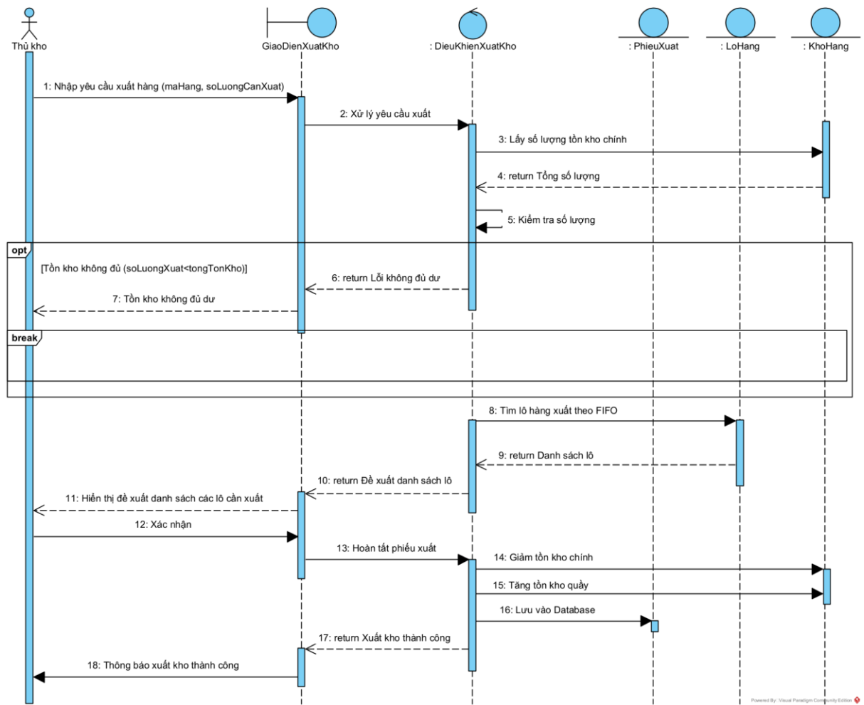
Hình 3.42. Biểu đồ tuần tự chức năng Xuất hàng ra quầy
