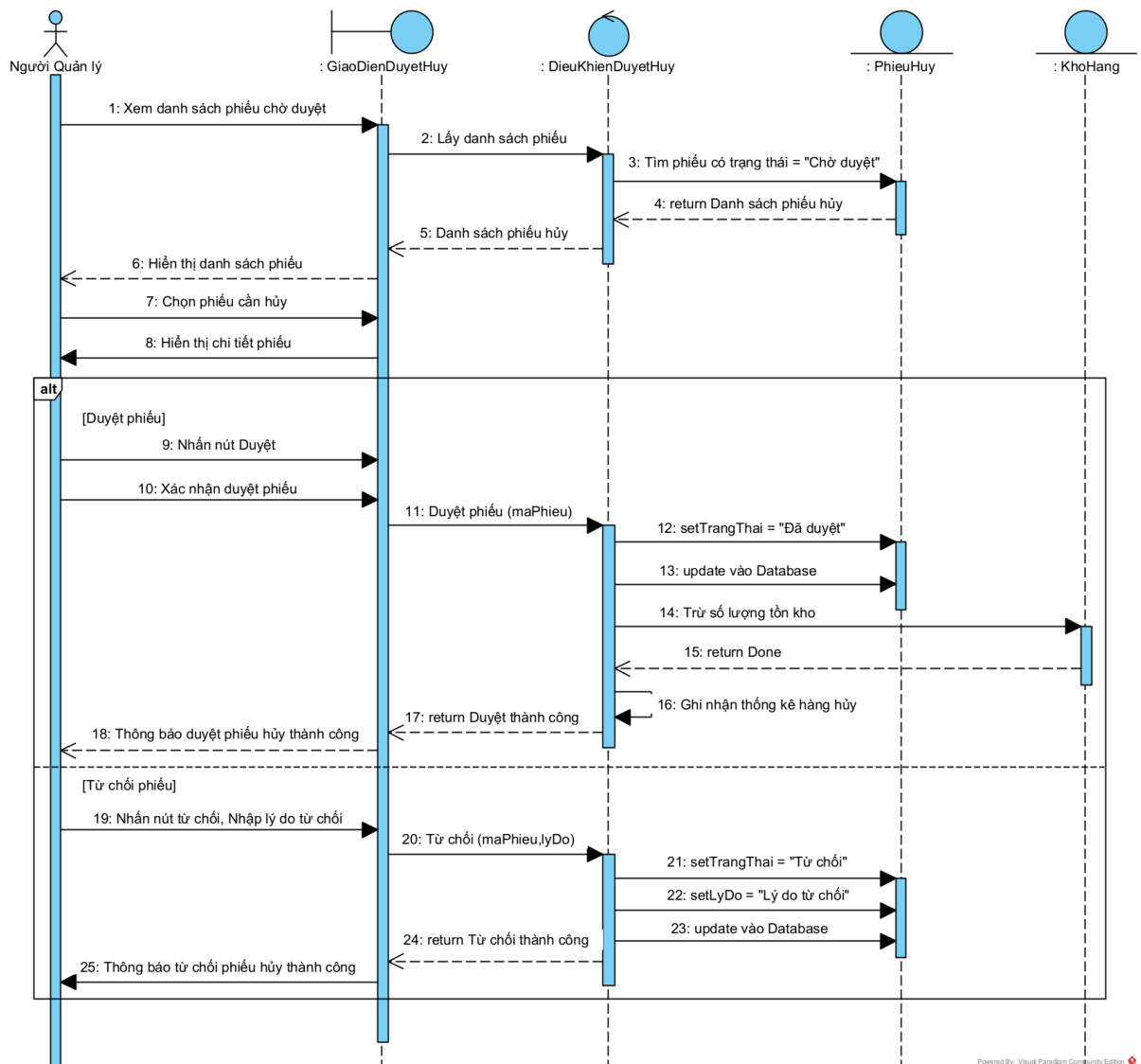
Hình 3.44. Biểu đồ tuần tự chức năng Duyệt phiếu hủy hàng
