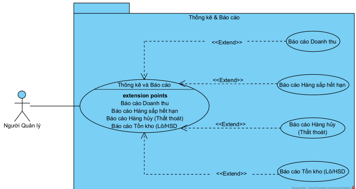
Hình 3.16. Biểu đồ UC mức 2 gói Thống kê và Báo cáo
