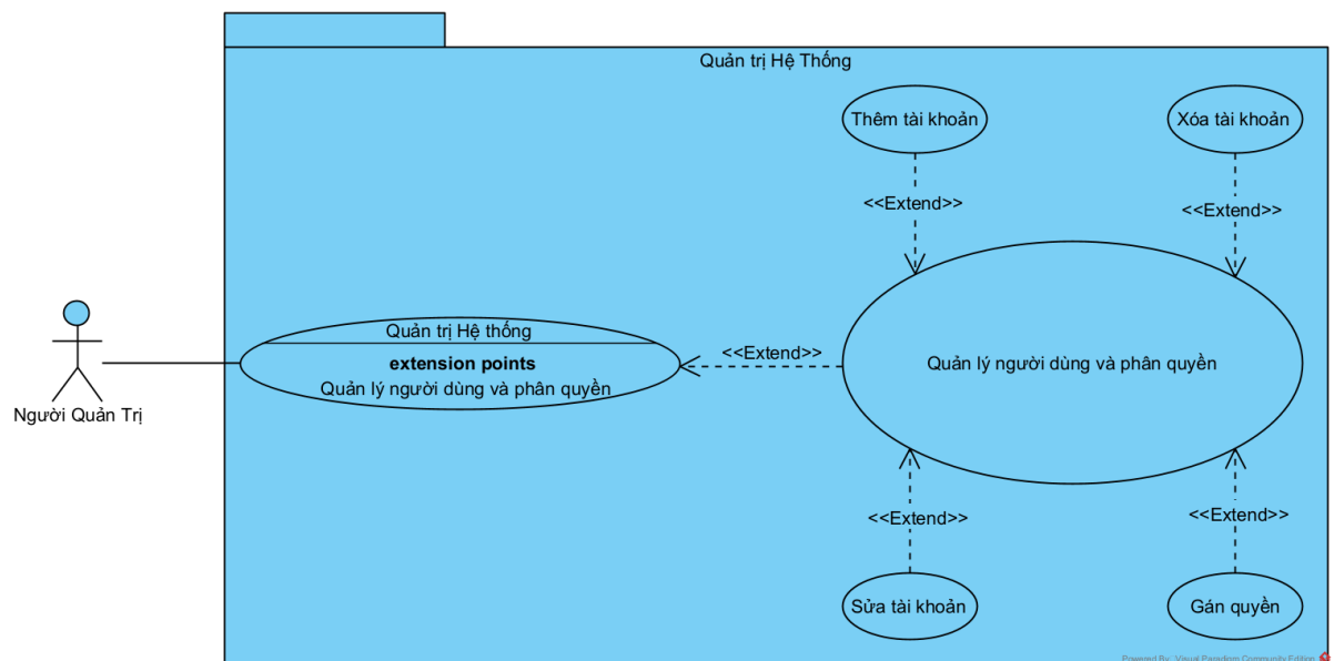
Hình 3.2. Biểu đồ UC mức 2 gói Quản trị hệ thống
