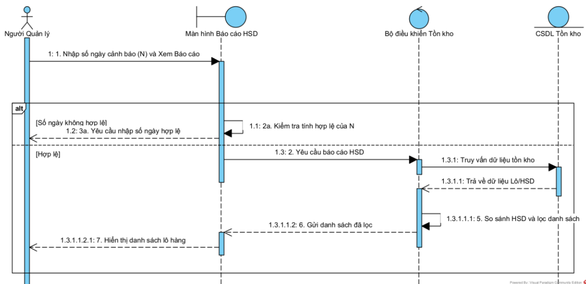
Hình 3.59. Biểu đồ tuần tự chức năng Báo cáo Hàng sắp hết hạn
