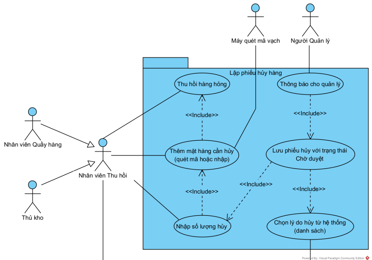
Hình 3.9. Biểu đồ UC mức 3 Lập phiếu hủy hàng
