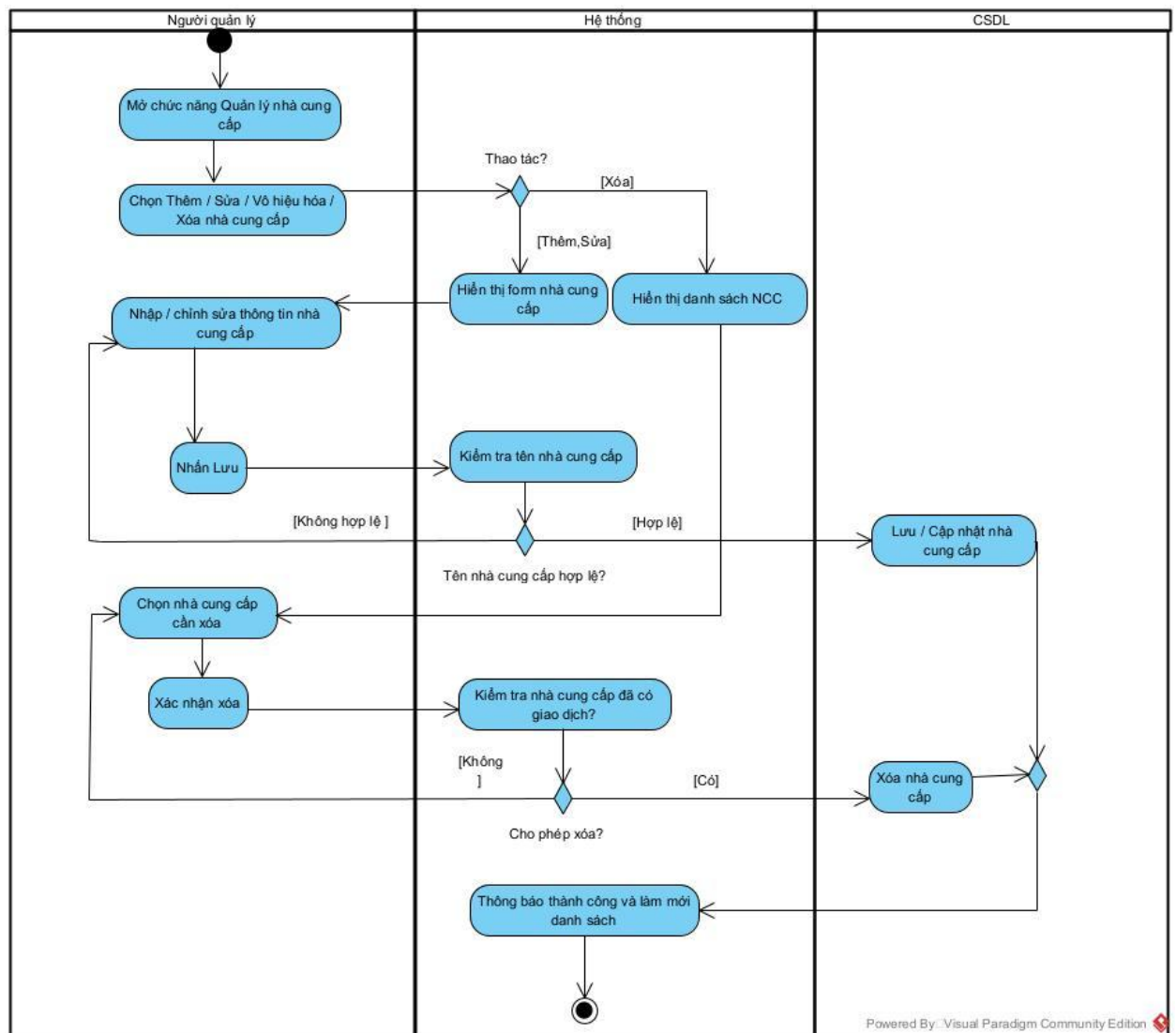
Hình 3.29. Biểu đồ Activity Quản lý nhà cung cấp
