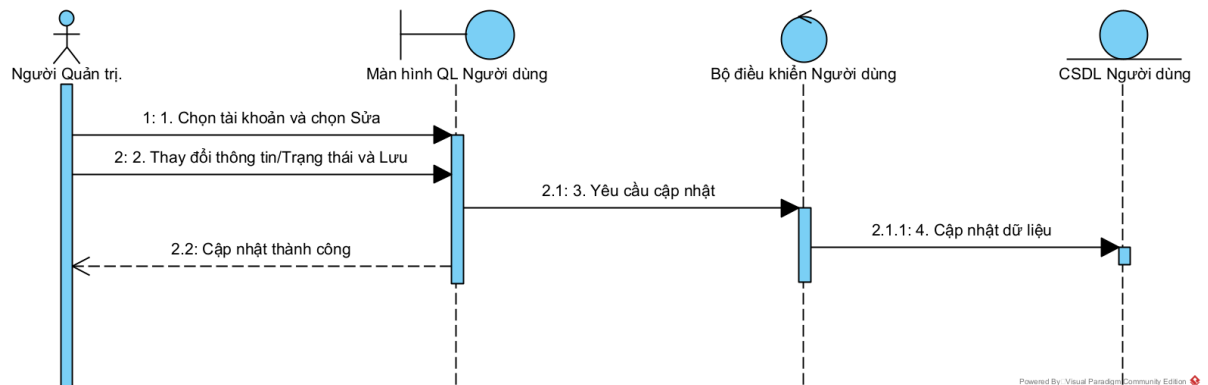
Hình 3.37. Biểu đồ tuần tự chức năng Sửa tài khoản
