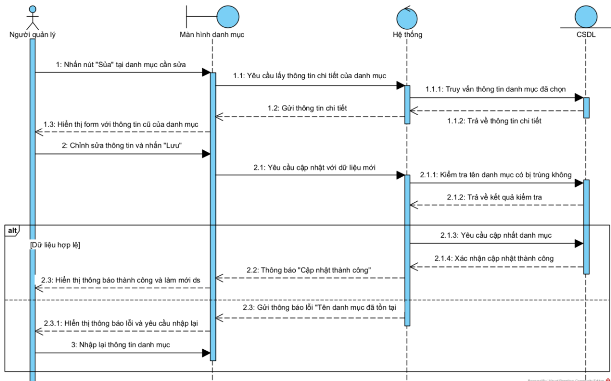
Hình 3.46. Biểu đồ tuần tự chức năng Sửa danh mục Ngành hàng
