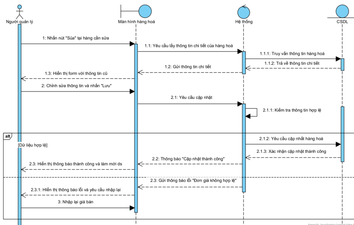
Hình 3.49. Biểu đồ tuần tự chức năng Sửa hàng hóa
