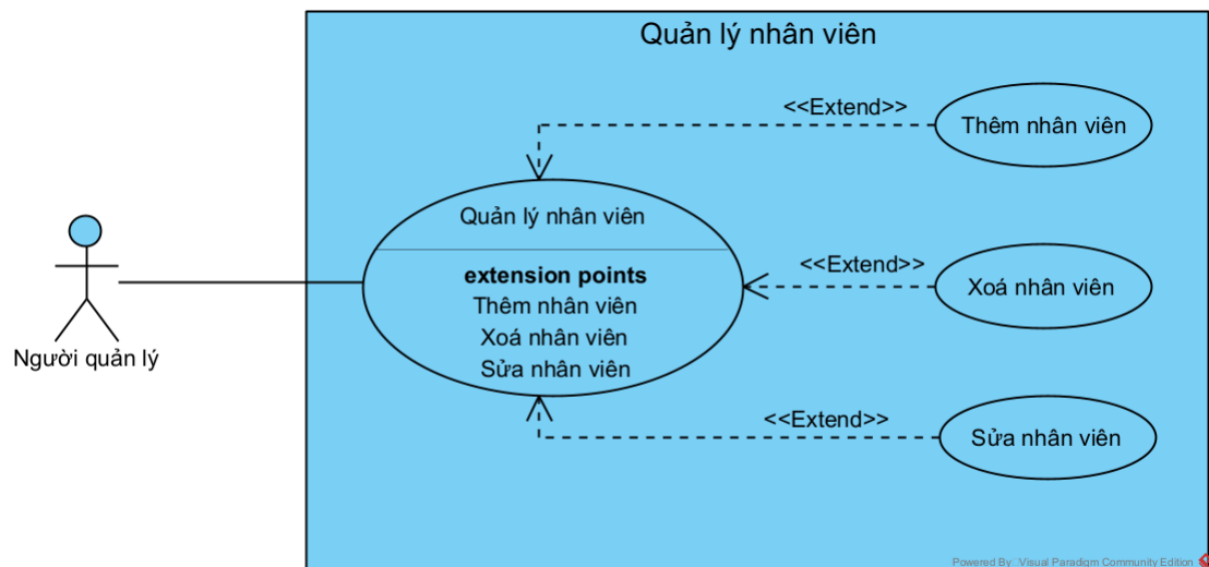
Hình 3.14. Biểu đồ UC mức 3 Quản lý nhân viên
