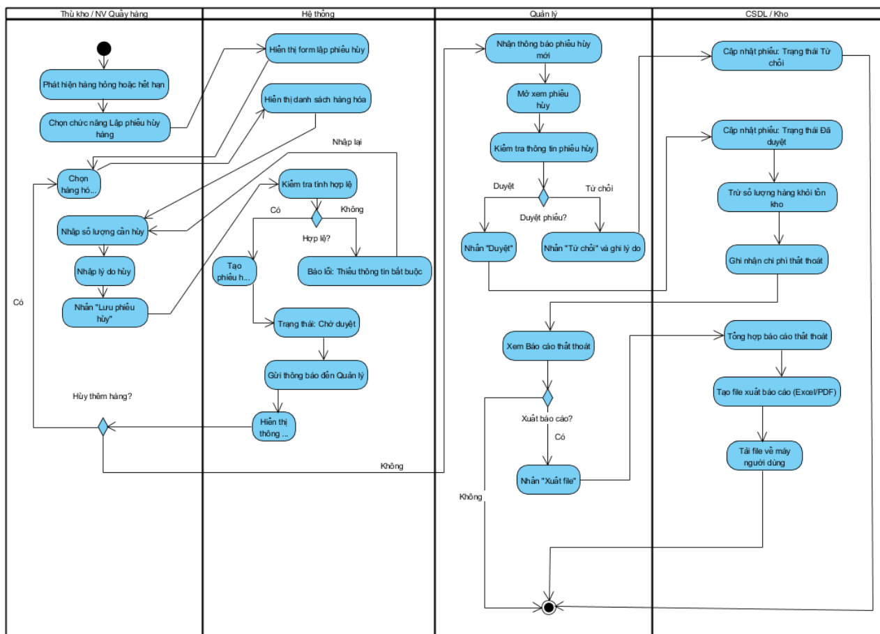
Hình 3.25. Biểu đồ Activity Hàng hủy và thất thoát
