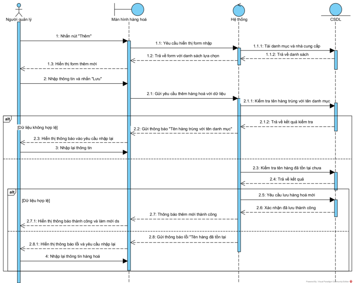
Hình 3.48. Biểu đồ tuần tự chức năng Thêm mới hàng hóa
