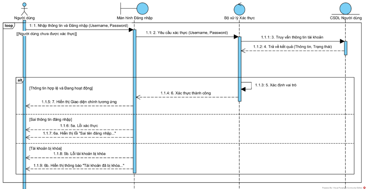
Hình 3.35. Biểu đồ tuần tự chức năng Đăng nhập
