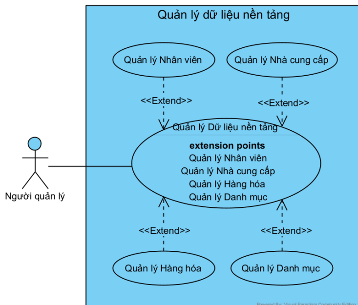
Hình 3.11. Biểu đồ UC mức 2 gói Quản lý Dữ liệu nền tảng
