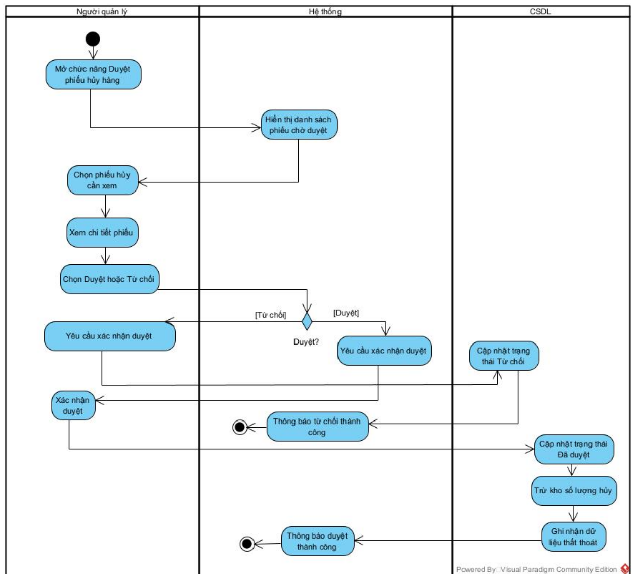
Hình 3.33. Biểu đồ Activity Duyệt phiếu hủy hàng
