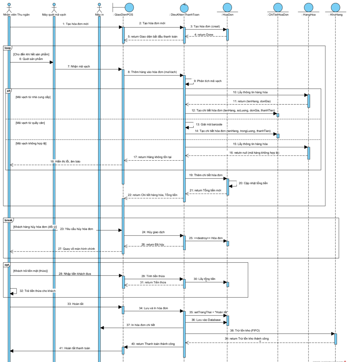
Hình 3.40. Biểu đồ tuần tự chức năng Thanh toán Hóa đơn
