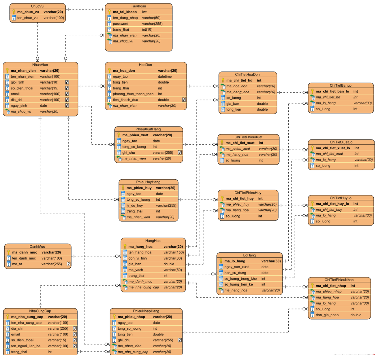
Hình 4.1. Biểu đồ ERD
