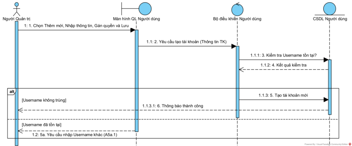
Hình 3.36. Biểu đồ tuần tự chức năng Thêm tài khoản
