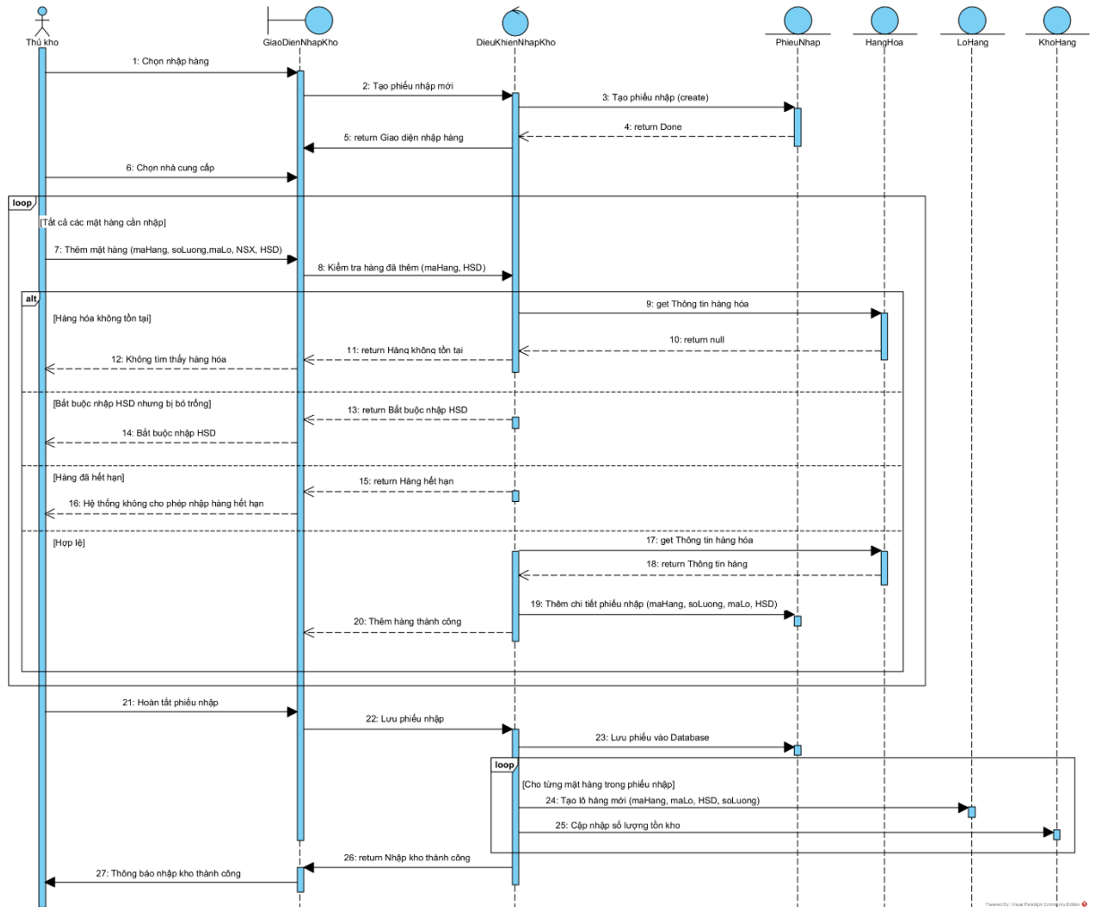
Hình 3.41. Biểu đồ tuần tự chức năng Nhập hàng vào kho
