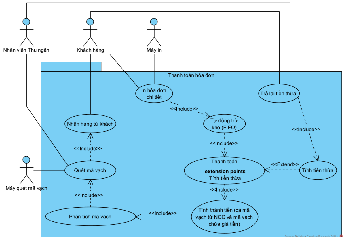
Hình 3.5. Biểu đồ UC mức 3 Thanh toán hóa đơn
