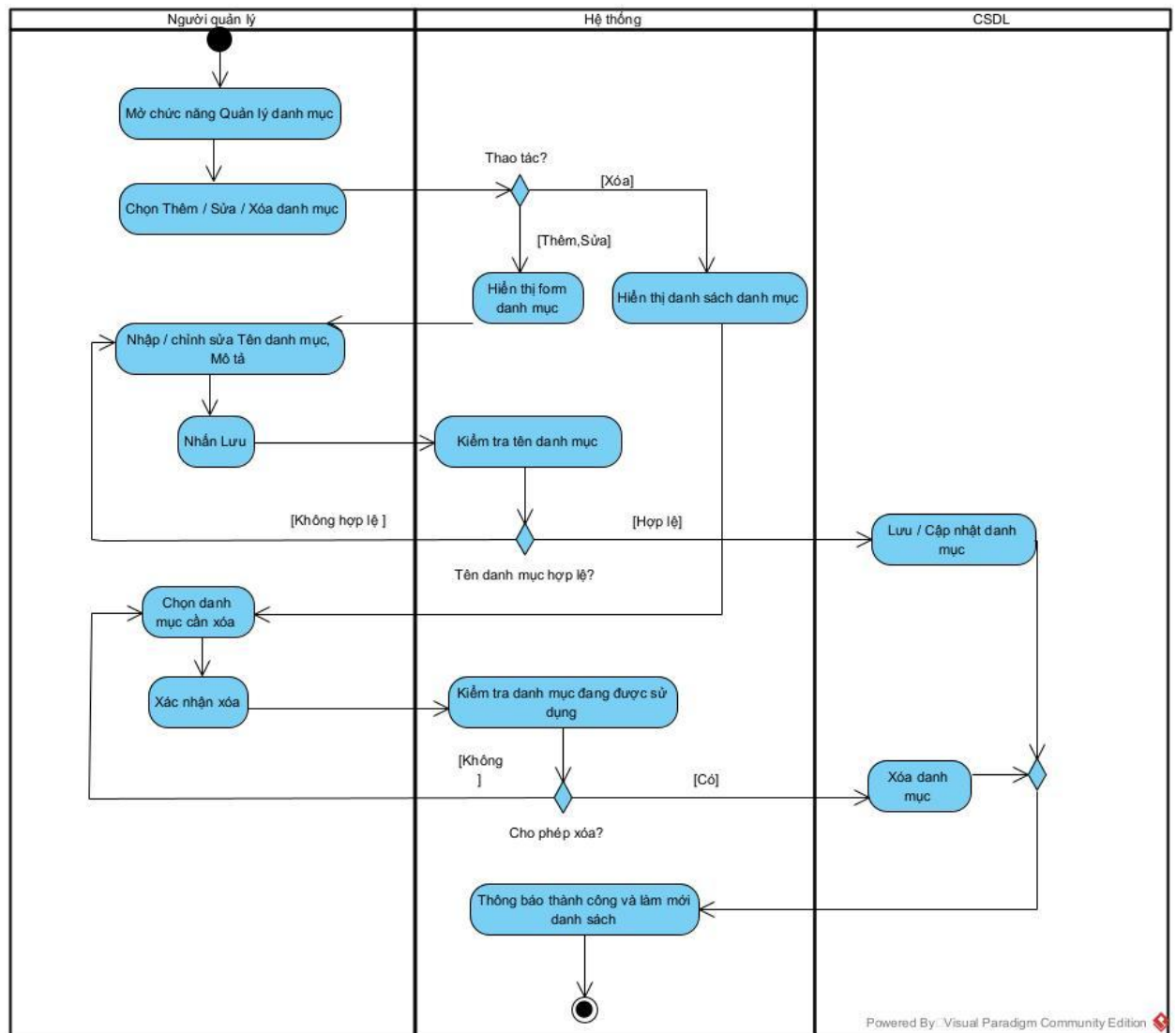
Hình 3.26. Biểu đồ Activity Quản lý danh mục
