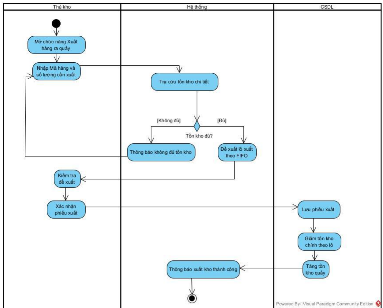
Hình 3.31. Biểu đồ Activity Xuất hàng ra quầy
