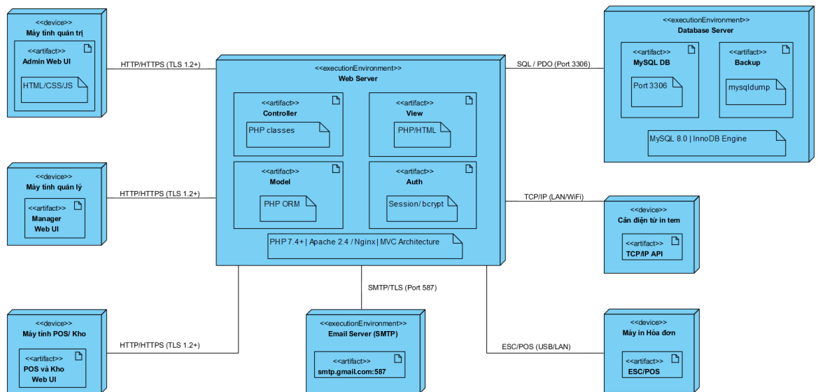
Hình 3.63. Biểu đồ Deployment
