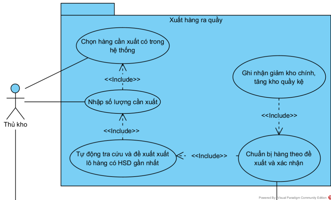
Hình 3.8. Biểu đồ UC mức 3 Xuất hàng ra quầy
