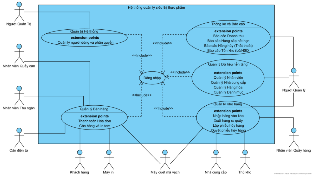
Hình 3.1. Biểu đồ UC Tổng quát
