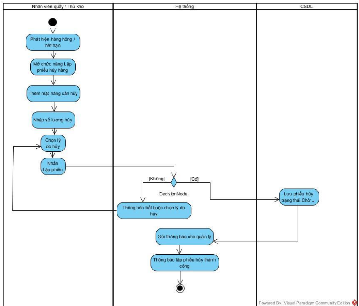
Hình 3.32. Biểu đồ Activity Lập phiếu hủy hàng
