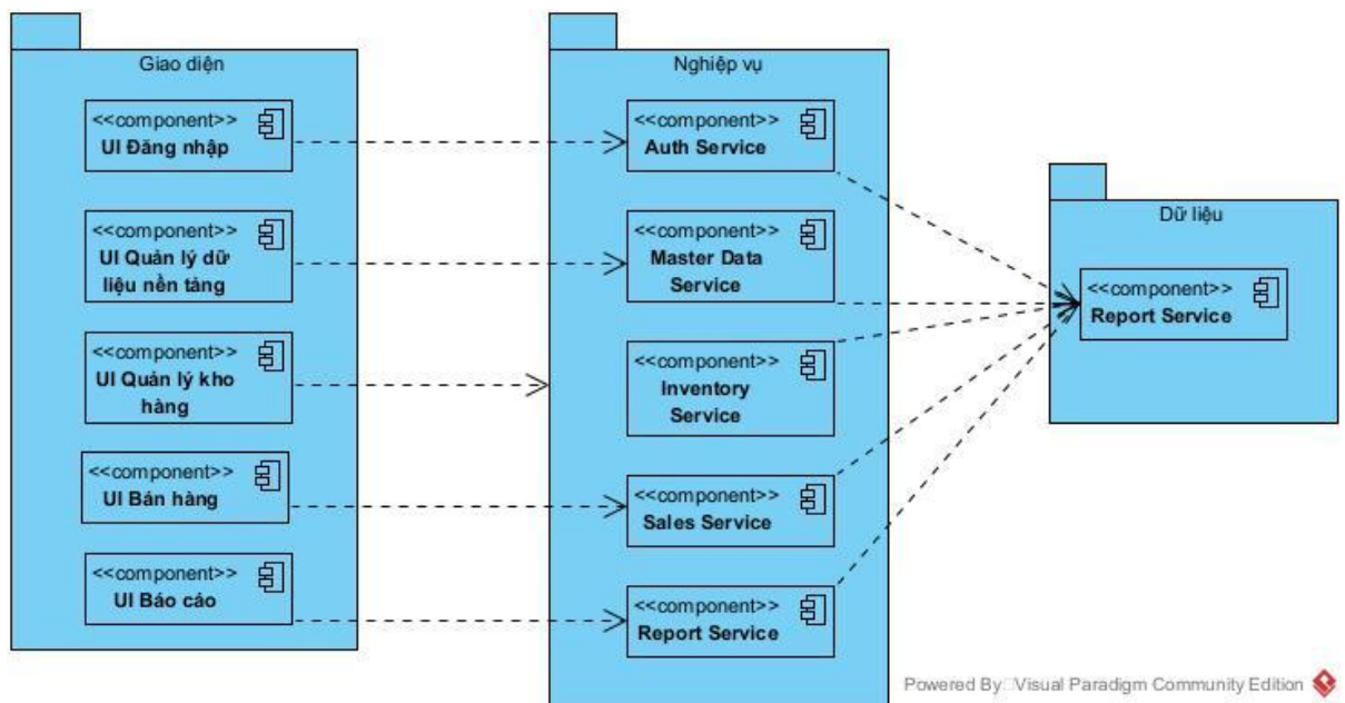
Hình 3.62. Biểu đồ Component
