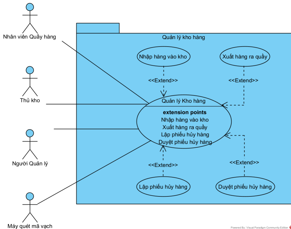
Hình 3.6. Biểu đồ UC mức 2 gói Quản lý kho hàng
