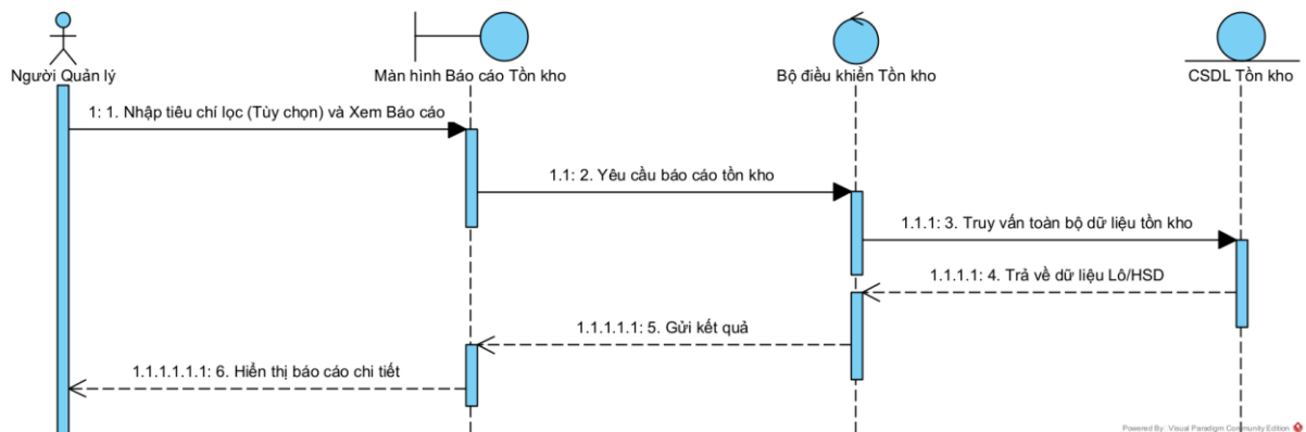
Hình 3.61. Biểu đồ tuần tự chức năng Báo cáo tồn kho
